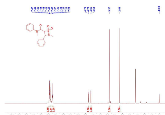
图 35 产物 3al 的核磁共振氢谱 Figure 35 ^1\text{H} NMR Spectrum of Product 3al
