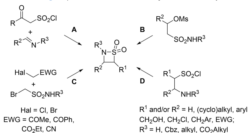
图4 \beta -磺内酰胺的经典合成方法
