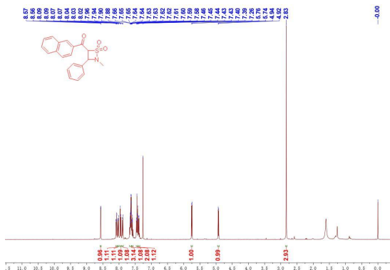
图 31 产物 3aj (萘-2-基) 的核磁共振氢谱 Figure 31 ^1\text{H} NMR spectrum of product 3aj (naphthalen-2-yl)
