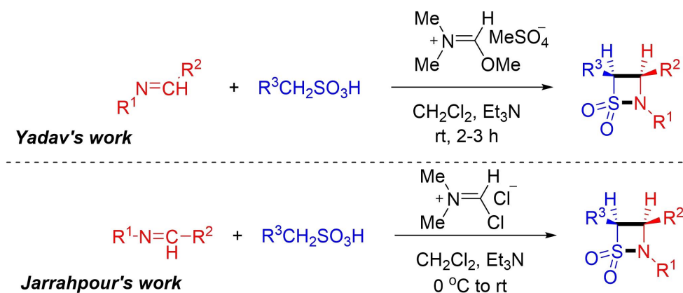
图6 Yadav 和 Jarrahpour 报道的 \beta -磺内酰胺合成方法
