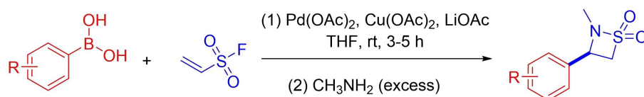
图5 \beta -芳基乙烯基磺酰氟的一锅法转化
