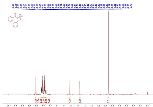
图 13 产物 3aa 的核磁共振氢谱 Figure 13 ^1\text{H} NMR Spectrum of Product 3aa
