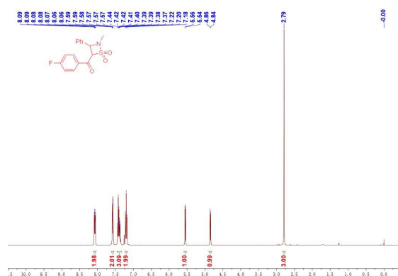
图 20 产物 3ad (4-氟苯基) 的核磁共振氢谱 Figure 20 ^1\text{H} NMR spectrum of product 3ad (4-fluorophenyl)
