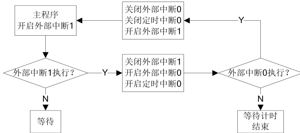
图 9 中断程序
